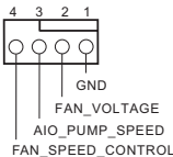
AIO_PUMP
